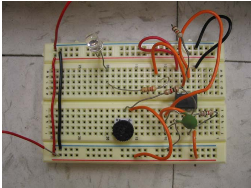
IR Circuit
